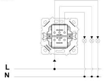
Bağlantı Şeması Connection Scheme Схема Подключения
