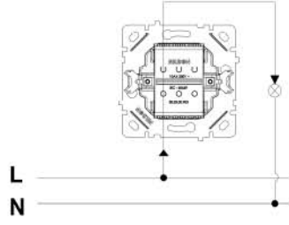
Bağlantı Şeması Connection Scheme Схема Подключения
