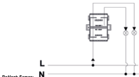
Bağlantı Şeması
