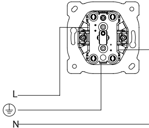
Bağlantı Şeması
