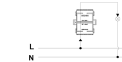
Bağlantı Şeması
